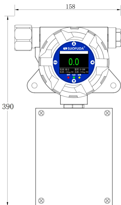
(图 1) 检测仪正视图
