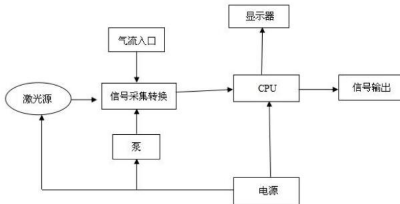
图 1、系统原理图
