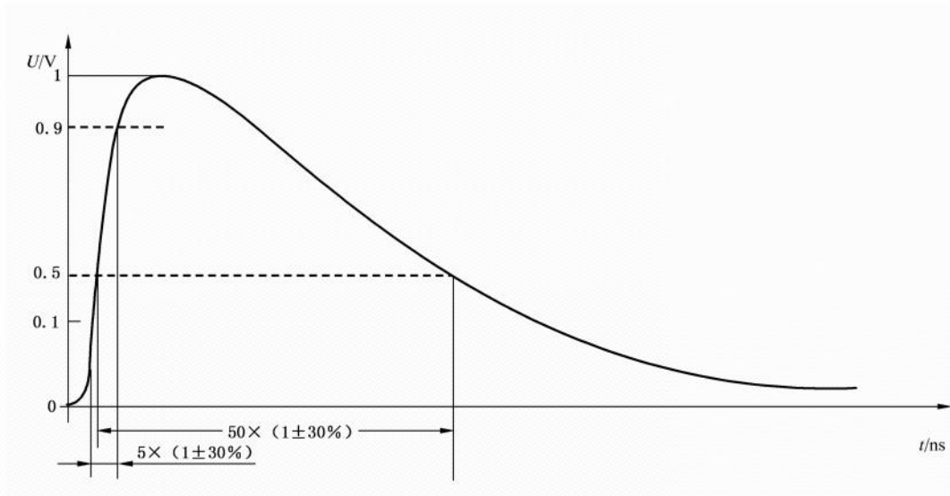
图 3 50Ω 负载时单脉冲波形
