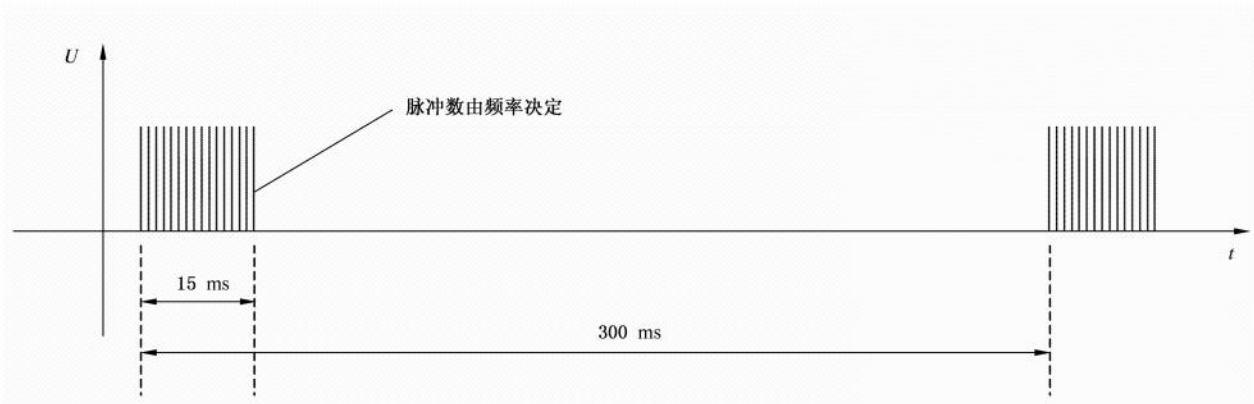
图 4 一组脉冲波形图
