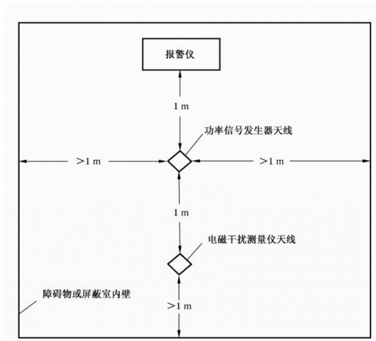
图 2 天线位置图
