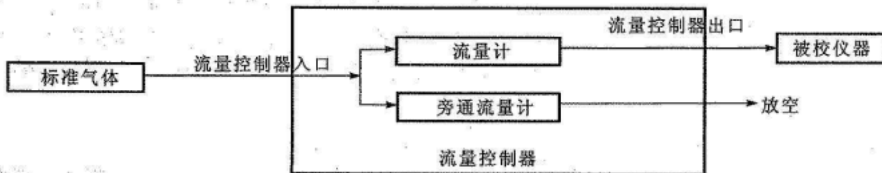
图1 仪器校准方框图
